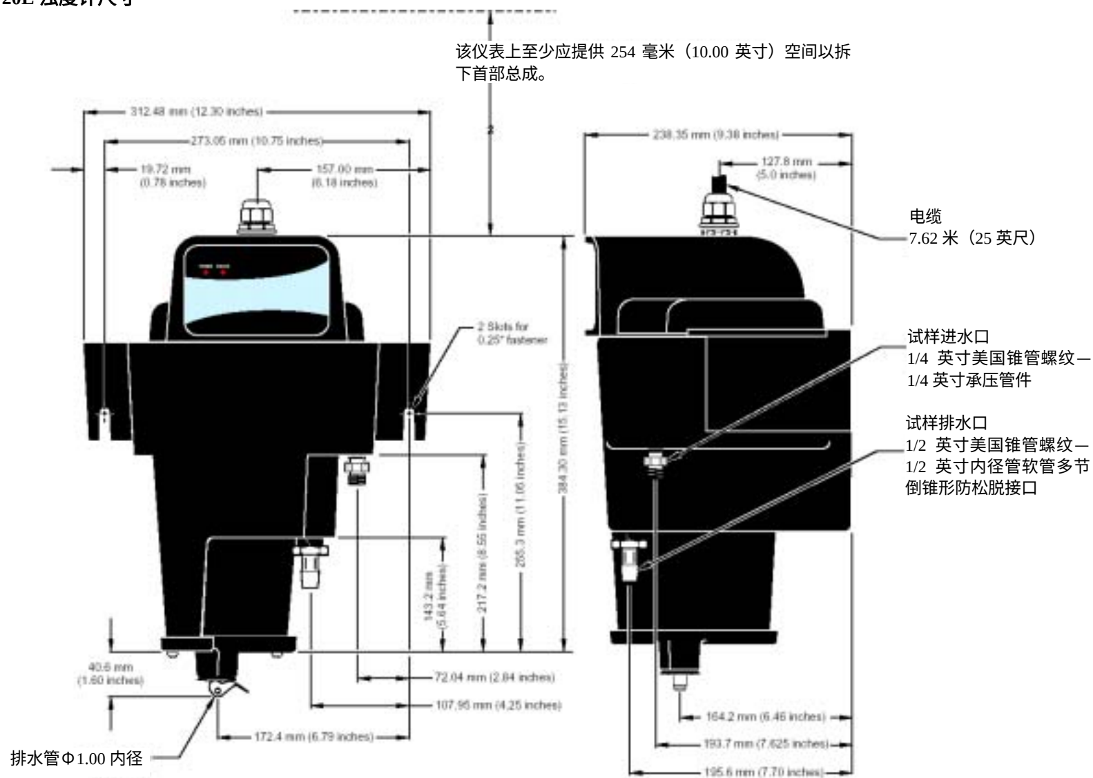
图 23 1720E 浊度计尺寸
